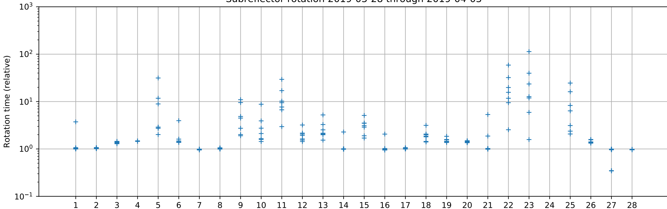
Subreflector rotation 2019-03-28 through 2019-04-03
